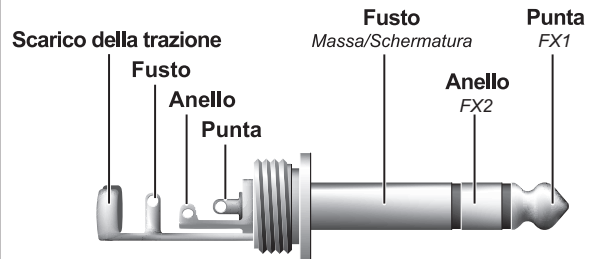
Fig. 5.5: Presse jack stereo per pedale
