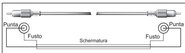
Fig. 5.3: Cavo RCA
