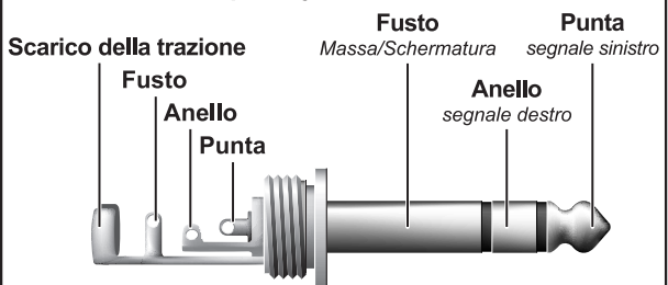
Fig. 5.6: Presse jack stereo per cuffia
