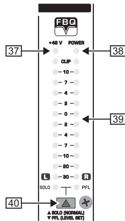
Fig. 2.16: Indicazione di livello
