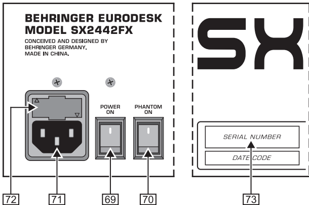
Fig. 2.28: Retro dell'EURODESK
