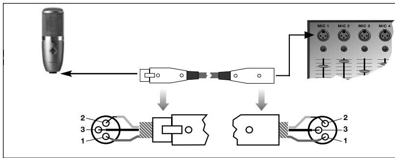
Fig. 3: Connexion sur une entrée symétrique avec alimentation fantôme.
